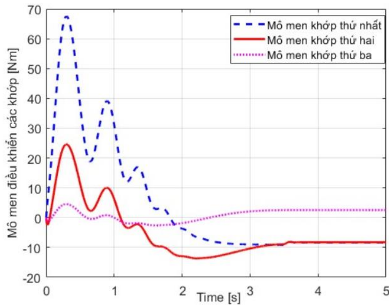
Mô men điều khiển các khớp cho robot Planar.
