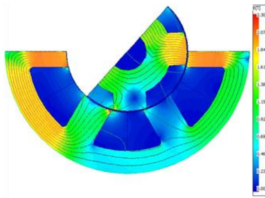
Mật độ từ cảm trên stator và rotor trong trường hợp góc cực \beta_s = 30^\circ ; \beta_r = 31^\circ .
