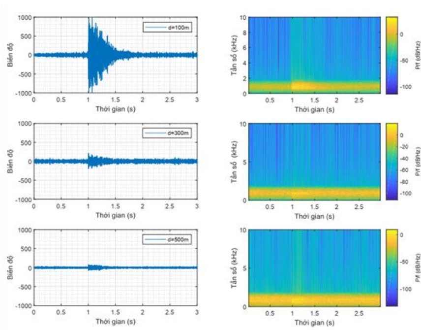
Tín hiệu âm thanh thu được sau bộ phân tích ICA tại các cự ly khác nhau.
