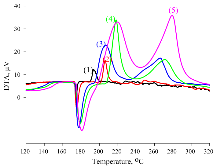
DTA curves of TNR at heating rates (1-2 \text{K}\cdot\text{min}^{-1} ; 2-5 \text{K}\cdot\text{min}^{-1} ; 3-10 \text{K}\cdot\text{min}^{-1} ; 4-10 \text{K}\cdot\text{min}^{-1} ; 5-20 \text{K}\cdot\text{min}^{-1} )
